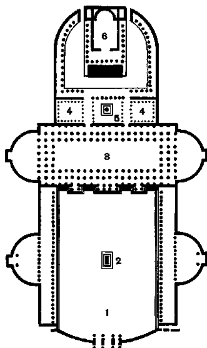
194 План форума императора Траяна: 1) Форум. 2) Конная статуя Траяна. 3) Базилика. 4) Библиотеки. 5) Колонна Траяна. 6) Храм Траяна
