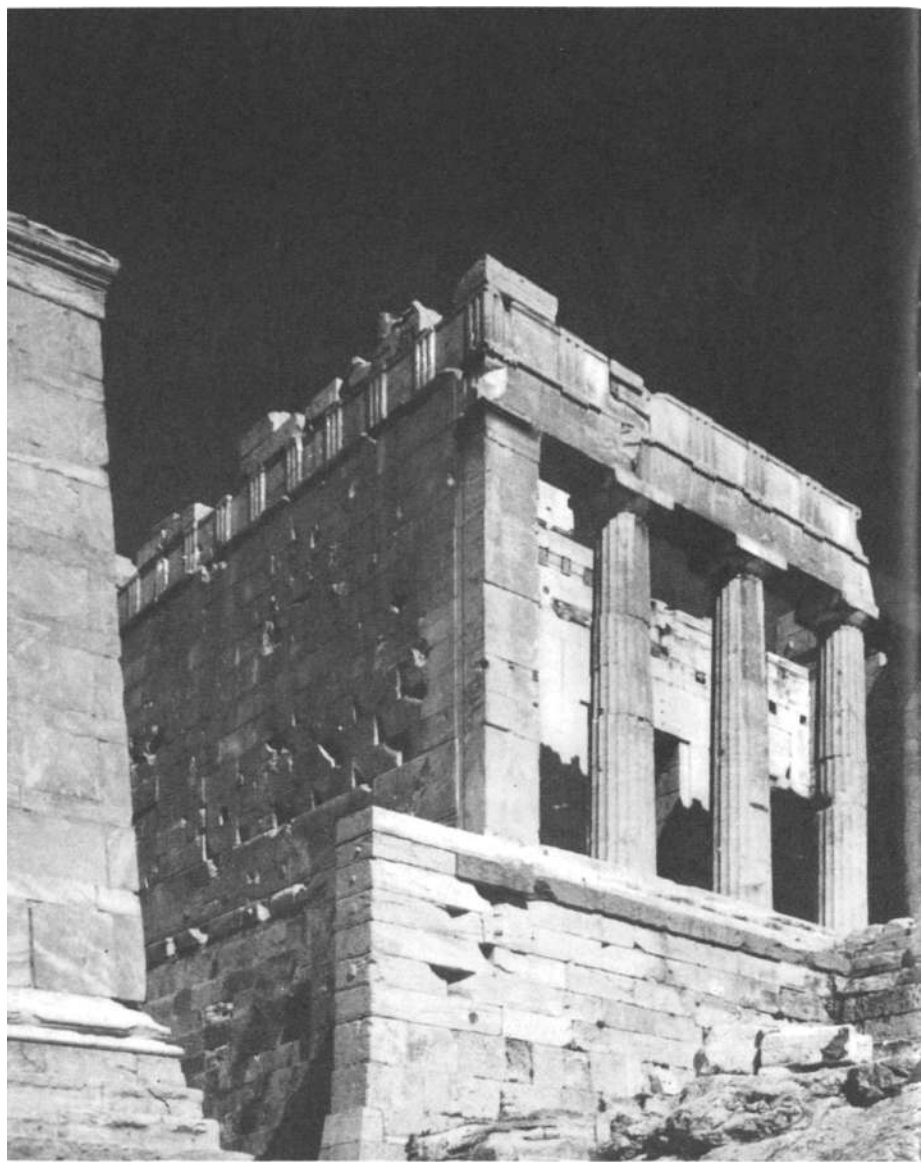
97 Архитектор Мнесикл. Пропилеи. Мрамор. 437—432 гг. до н. э. Афинский акрополь
